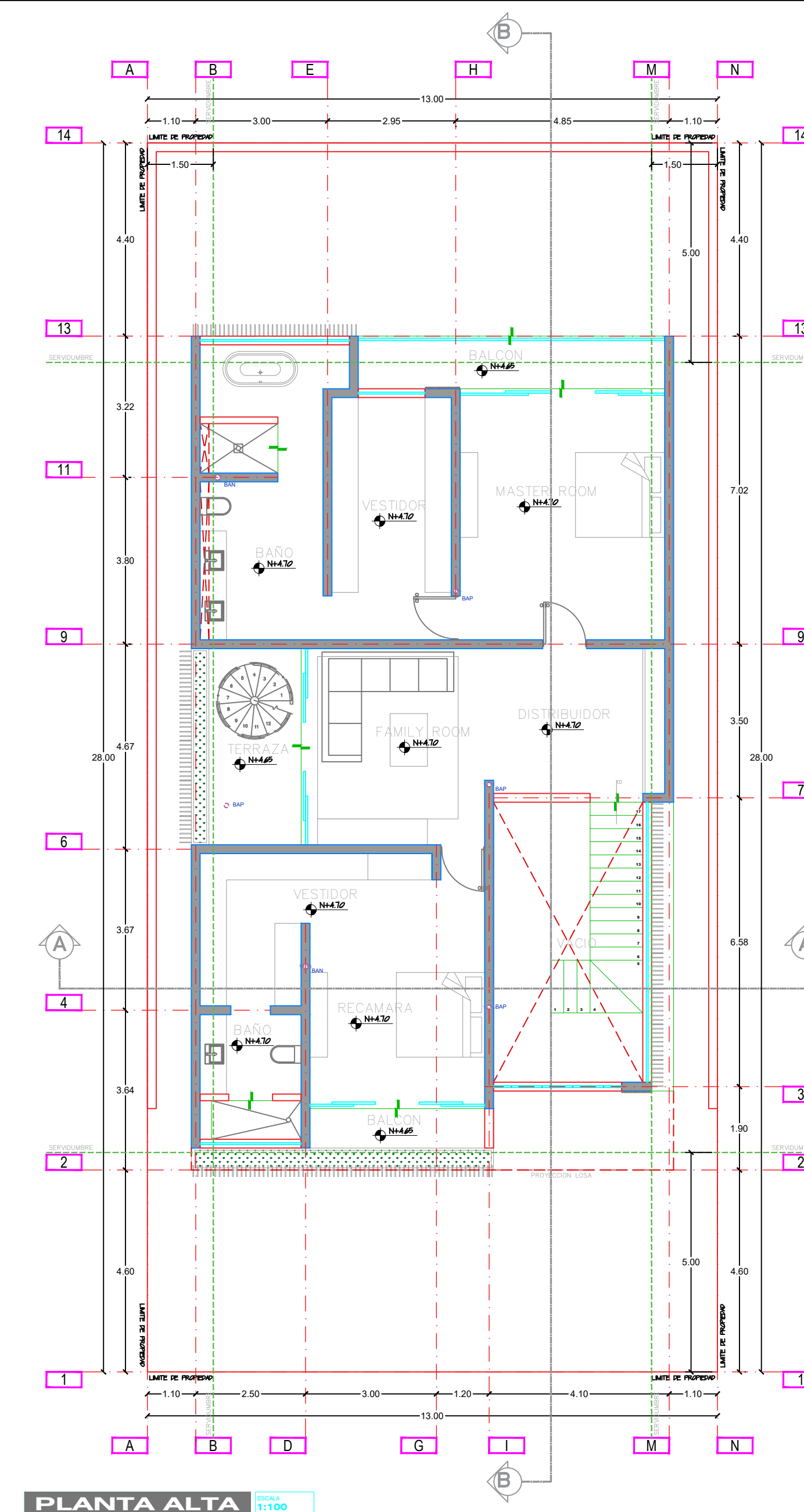
PLANTA ALTA ESCALA 1:100
