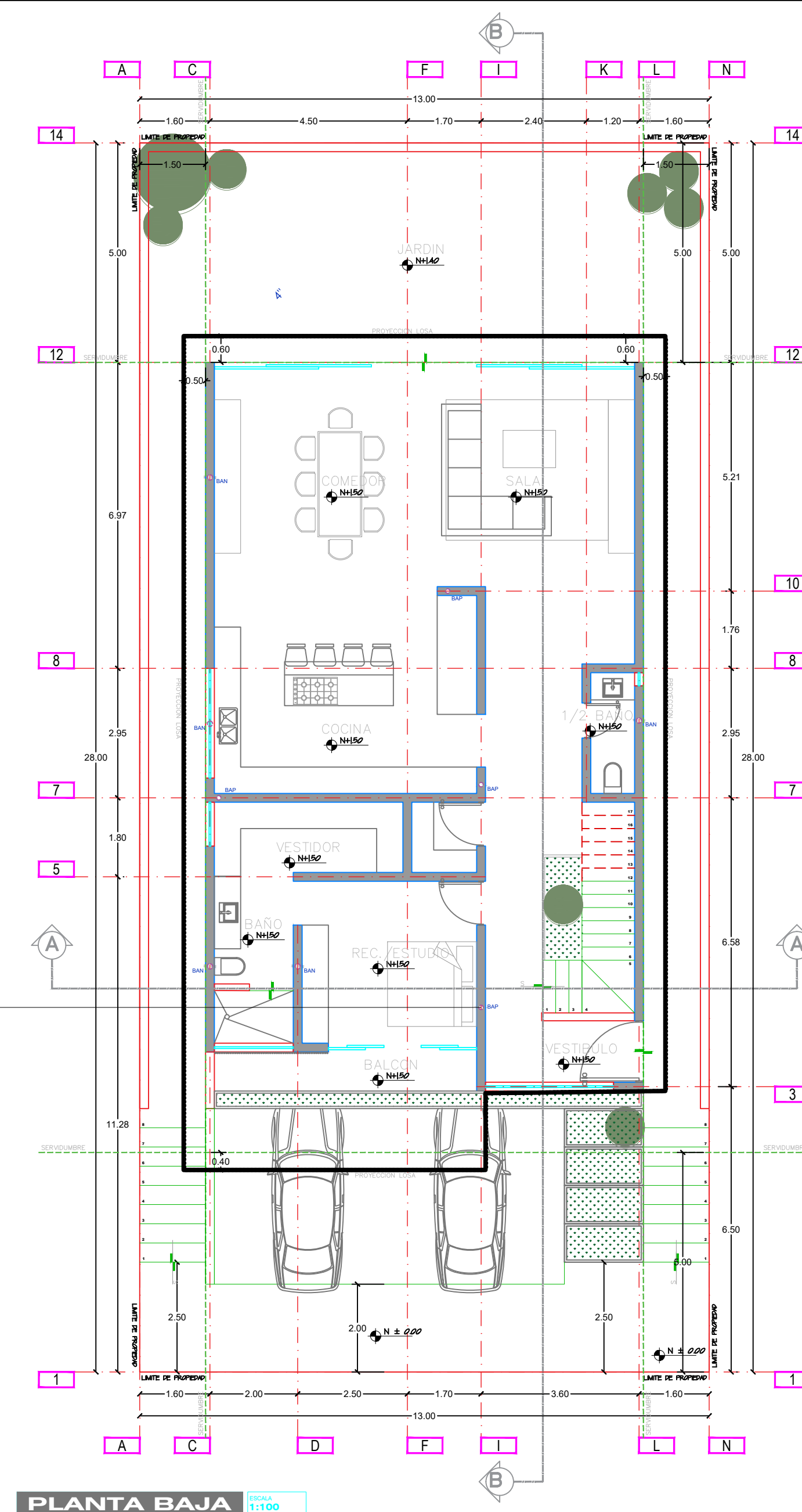
PLANTA BAJA ESCALA 1:100
