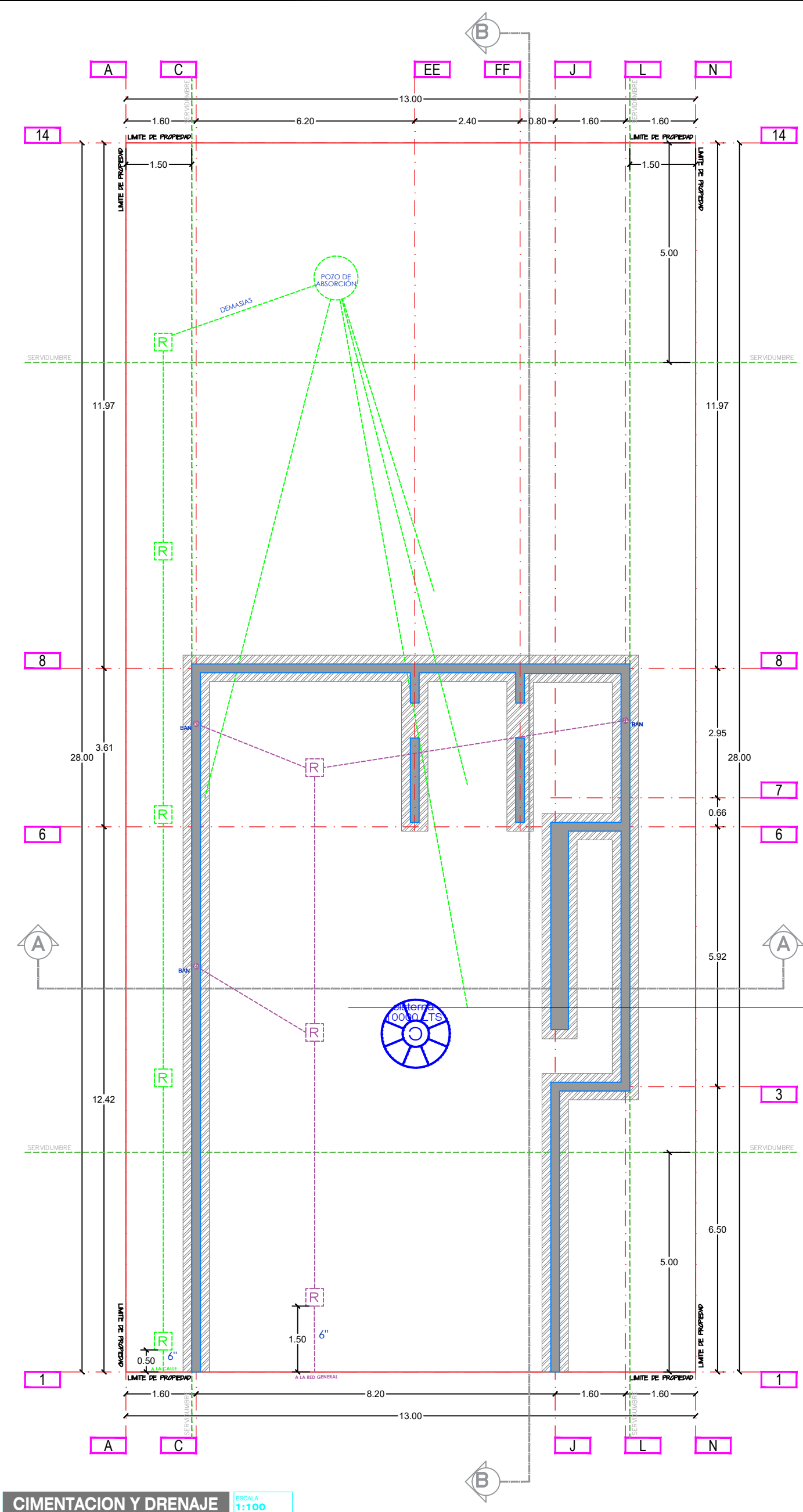
CIMENTACION Y DRENAJE ESCALA 1:100
