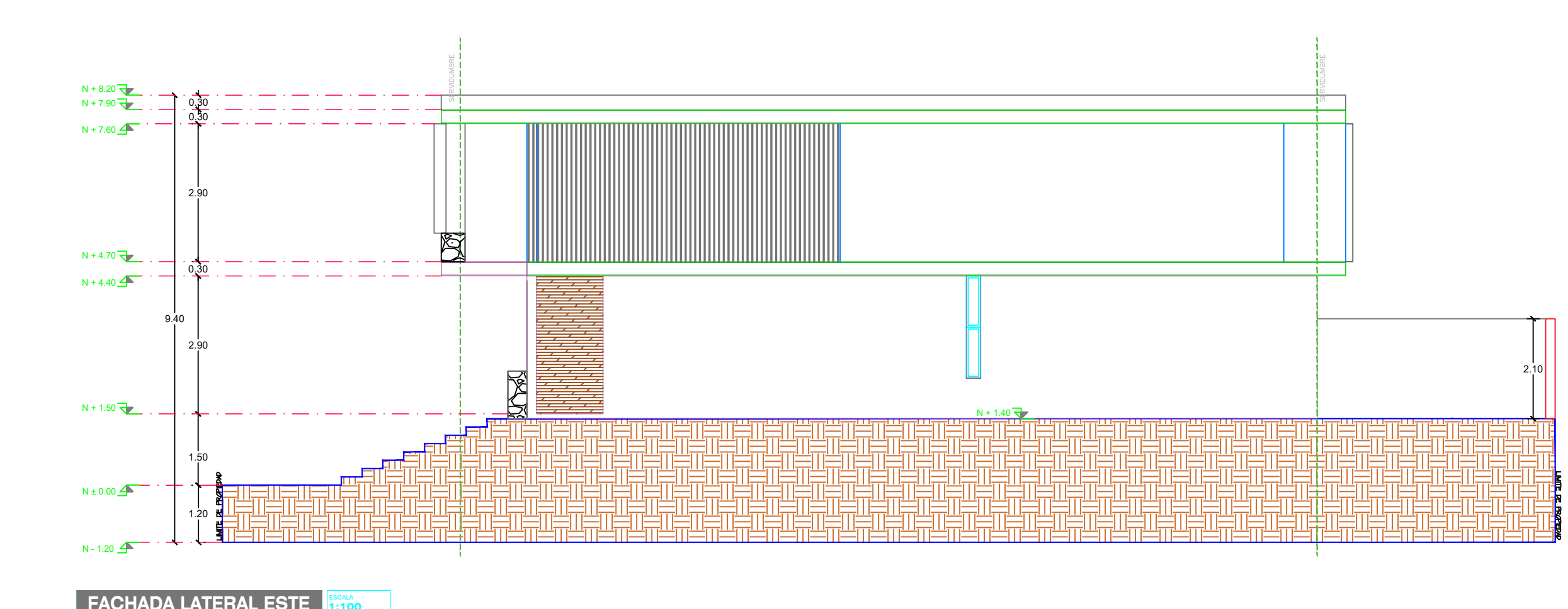
FACHADA LATERAL ESTE ESCALA 1:100
