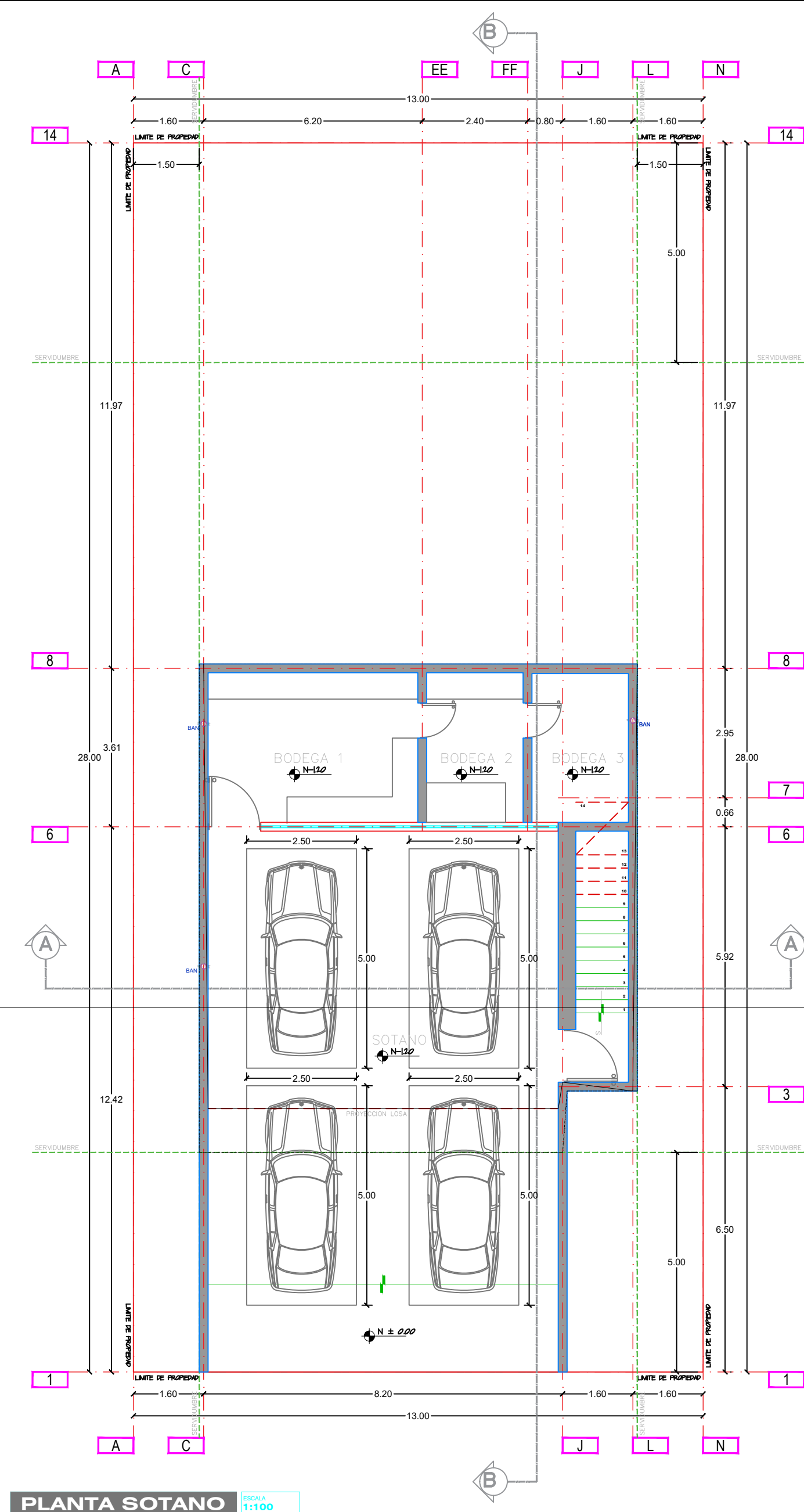
PLANTA SOTANO ESCALA 1:100
