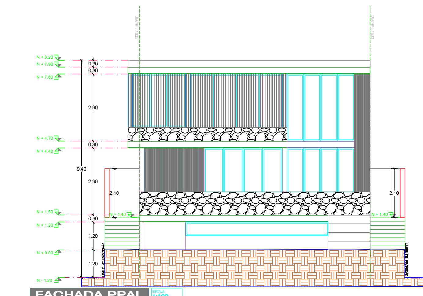
FACHADA PPAL ESCALA 1:100
